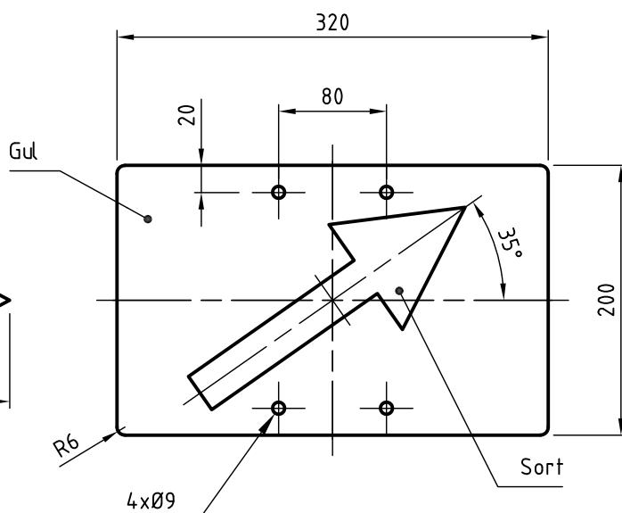
Utf. 1 Spor til høyre. Artikkelnr.: 114 107
